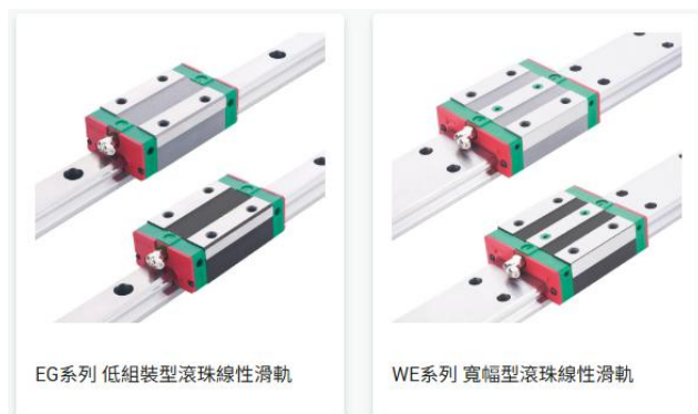
圖三、線性滑軌
